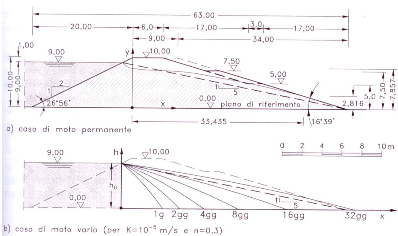
Figura 7-2 – Linea di infiltrazione a moto permanente (caso a) e a moto vario (caso b) di una arginatura (DA DEPPO et al., 2002; pag. 477).
