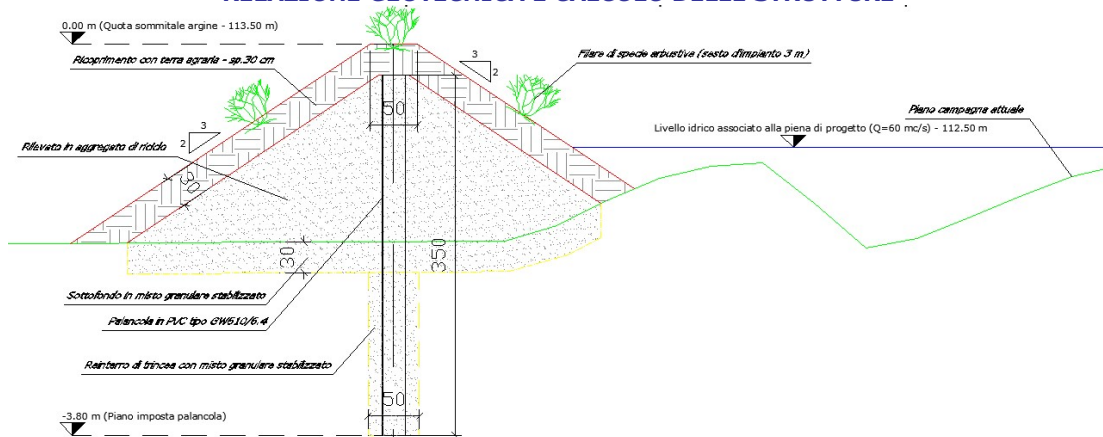
Figura 7-3: Schema di progetto del rilevato di presidio
