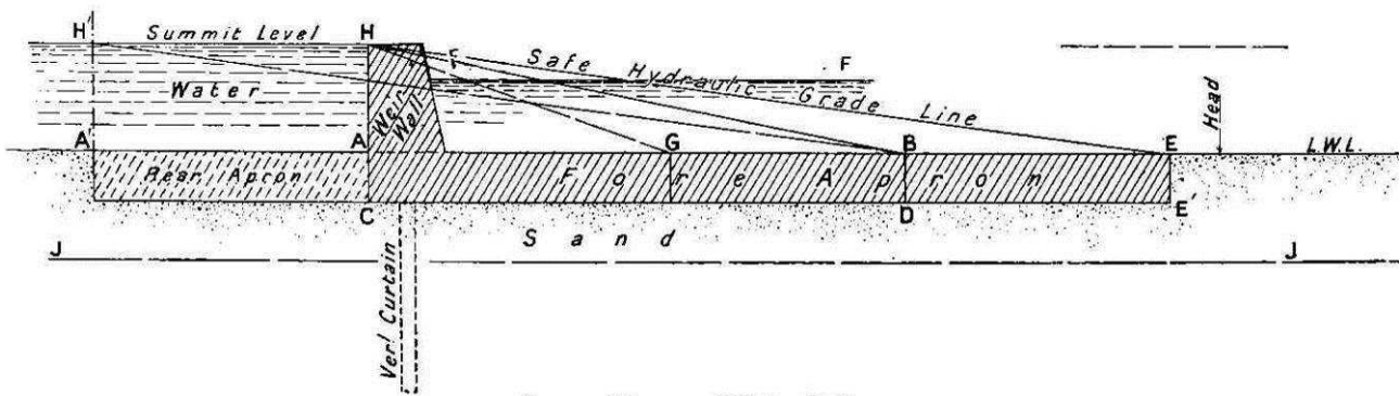
Figura 7-1 Schema di traversa in cui Bligh introduce la linea dei carichi (seconda edizione del 1910; pag. 165).
