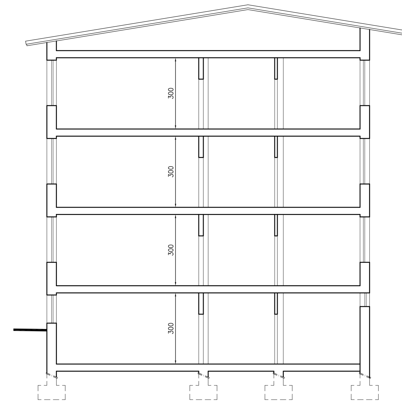
SEZIONE TRASVERSALE SCUOLA SECONDARIA Scala 1:100
