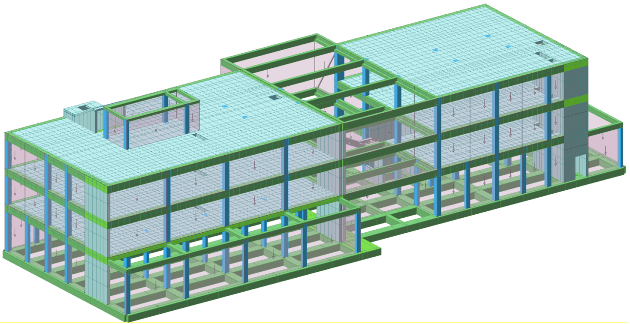
Vista modello strutturale lato Est
