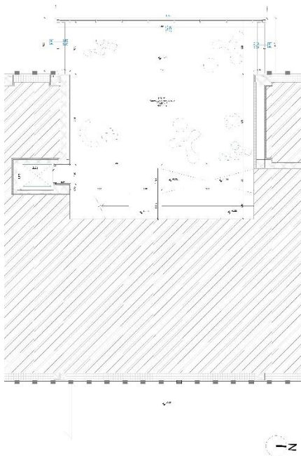
Pianta pianerottolo panoramico
