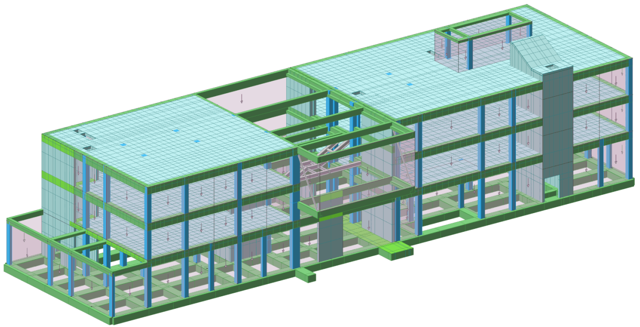
Vista modello strutturale lato Ovest
